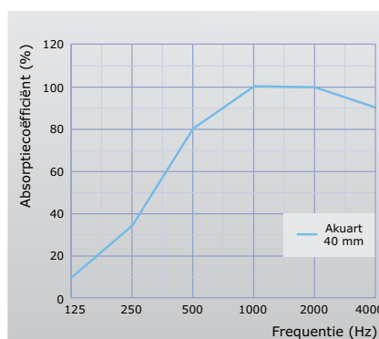
Geluidsabsorptiewaarden
