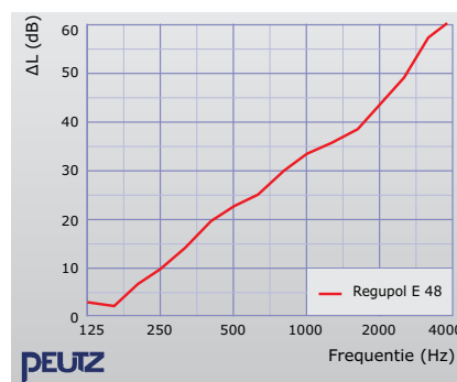
Contactgeluidisolatieverbetering \Delta L
